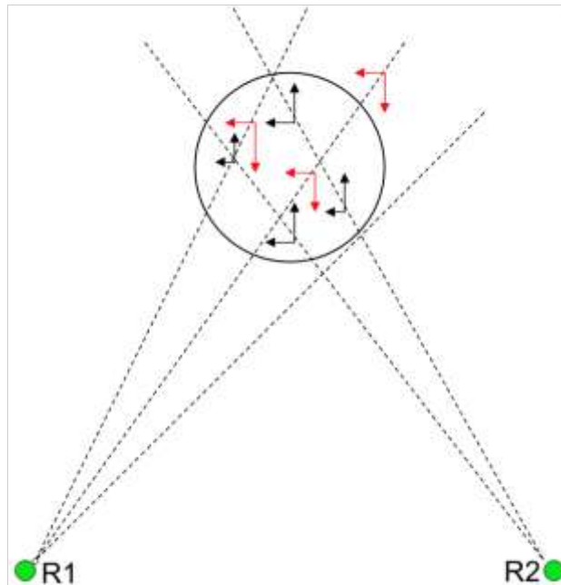
Slika 1.8.8.2. Izračun brzine i smjera struja u predefiniranom krugu oko točke mreže, na temelju radialnih mjerenja postaja VF radara R1 i R2.
