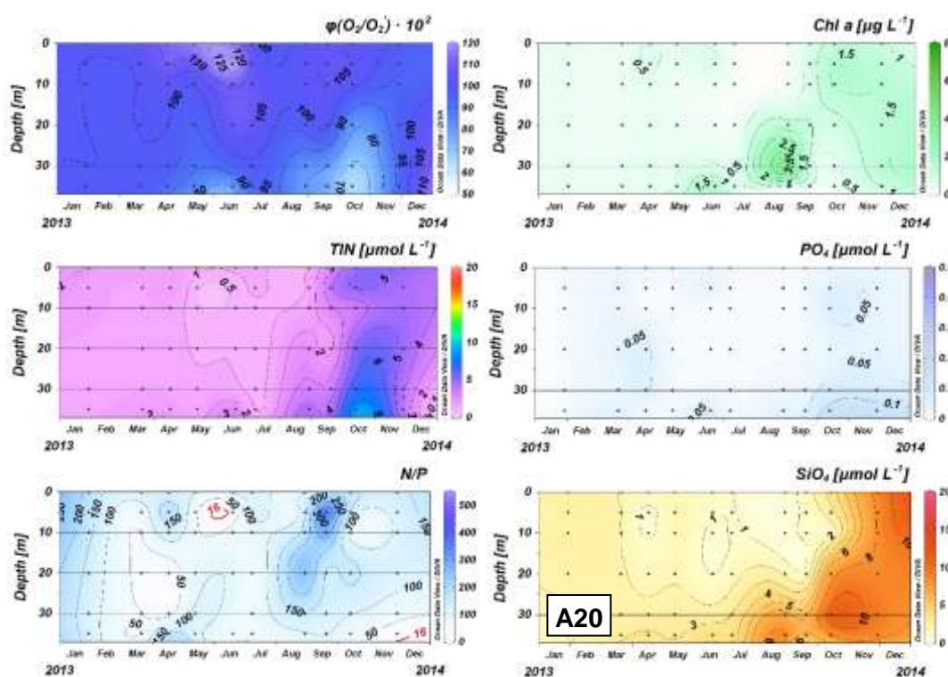
Slika 1.6.2. Raspodjela udjela zasićenja kisika ( \varphi(O_2/O_2') ), koncentracije klorofila a (Chl a), ukupnog otopljenog anorganskog dušika (TIN), ortofosfata ( PO_4 ) i ortosilikata ( SiO_4 ), i N/P omjera s dubinom na postaji A20 tijekom 2013.
