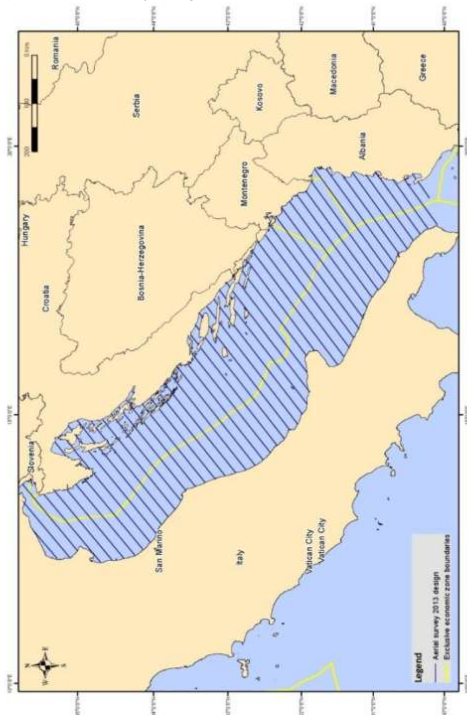
Slika 1.2.1. Odabrani transekci za monitoring brojnosti i rasprostranjenosti dobrih dupina i prugastih dupina u Jadranu
