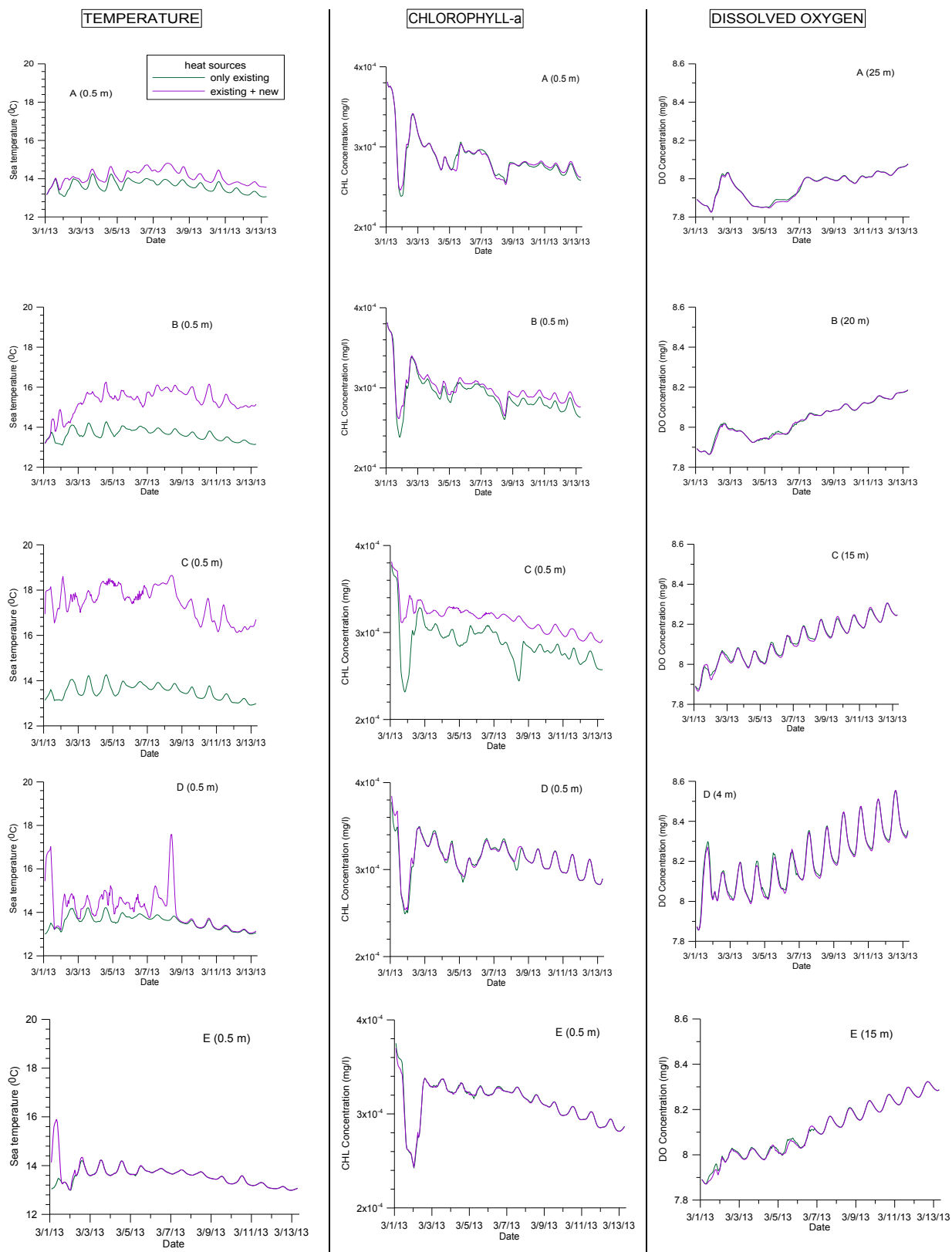
Slika 2.2.5. Temperatura mora na dubini 0.5m, koncentracija klorofila-a na dubini 0.5 m i koncentracija otopljenog kisika (dubine na grafovima) na točki A, B, C, D i E modela (dubine redom 25m, 20m, 15m, 4m i 15m, svi su nizovi 5-satni srednjaci).
