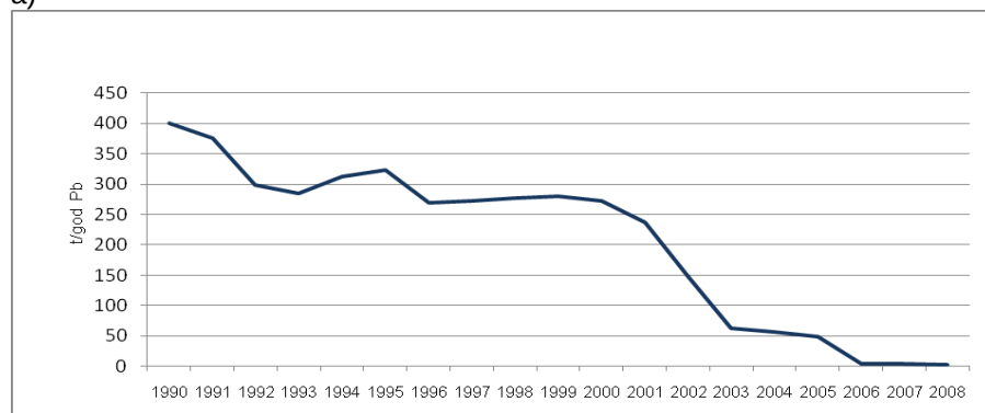
Slika 1.6. a) Emisije Pb. i b) Doprinis pojedinih sektora emisiji Pb
