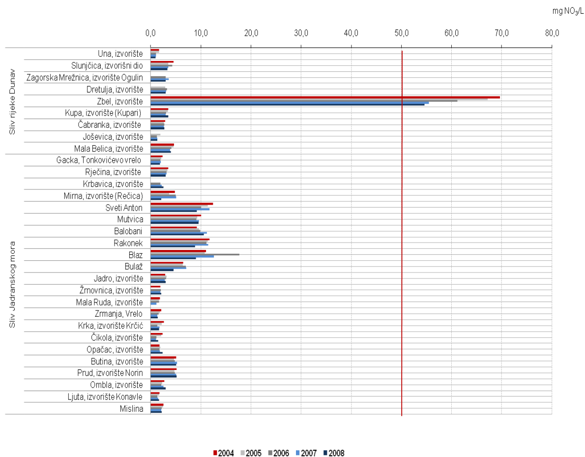
Slika 3.17. Srednje godišnje vrijednosti nitrata u izvorima
