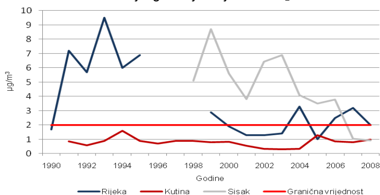
Slika 1.14. Trend srednjih godišnjih vrijednosti \text{H}_2\text{S}
