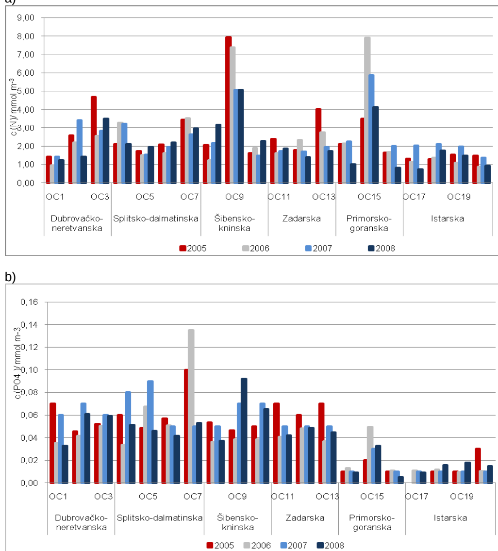
Slika 4.6. Srednje godišnje koncentracije hranjivih soli u sloju 0–10 m : a) N i b) \text{PO}_4^{3-}
