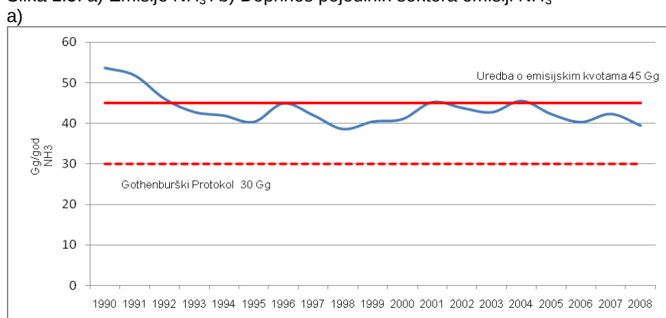
Slika 1.5. a) Emisije NH 3 i b) Doprinos pojedinih sektora emisiji NH 3
