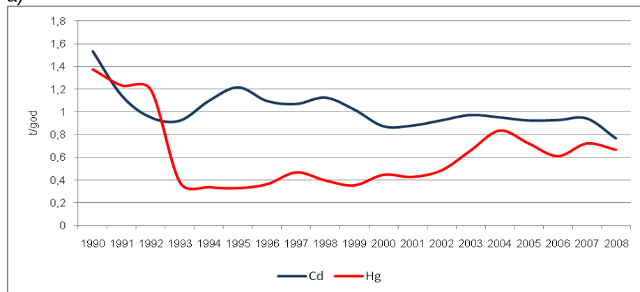
Slika 1.7. a) Emisije Hg i Cd i b) Doprinis pojedinih sektora emisiji Hg i Cd
