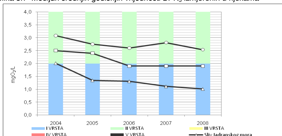
Slika 3.7 Medijan srednjih godišnjih vrijednosti BPK 5 izmjerenih u rijekama
