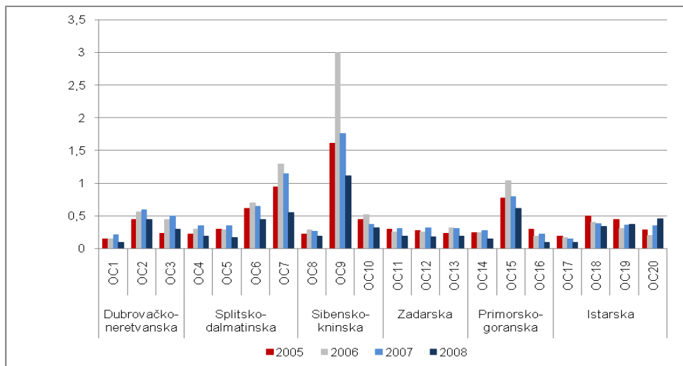
Slika 4.7. Srednje godišnje koncentracije klorofila a u površinskom sloju vodenog stupca (0 do 10 m)
