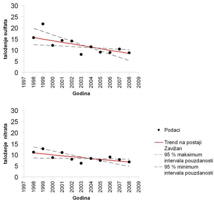
Slika 1.11. Trend taloženja sulfata i nitrata (kg/ha) za postaju Zavižan za razdoblje od 1997. do 2008. godine. Trend je određen Mann-Kendall testom, a nagib trenda Senovom neparametarskom metodom (Gillbert, 1987).
