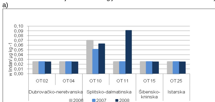
Slika 4.16. Maseni udjeli kloriranih ugljikovodika u morskom sedimentu: a) lindan, b) DDT, c) PCB
