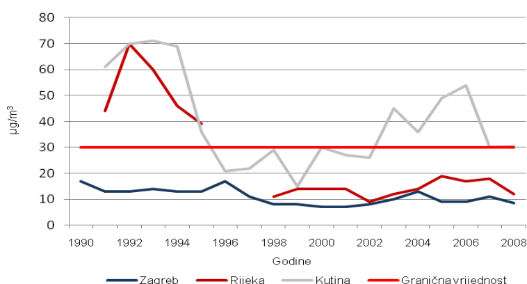
Slika 1.15. Trend srednjih godišnjih vrijednosti \text{NH}_3
