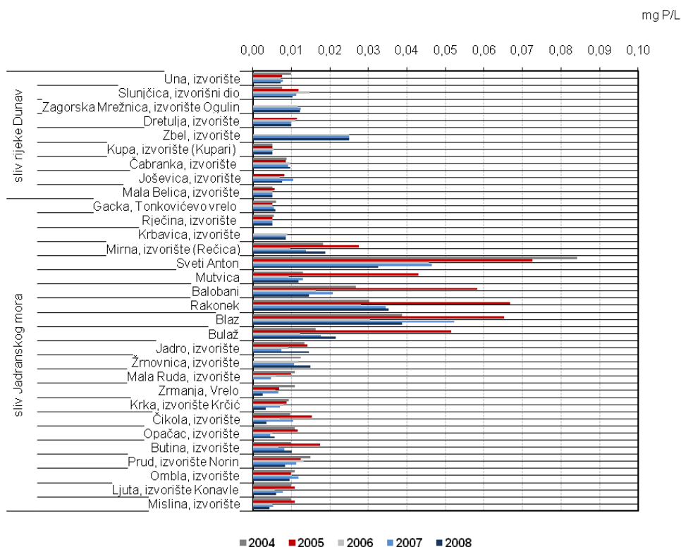
Slika 3.18. Srednje godišnje vrijednosti koncentracije ortofosfata u izvorima
