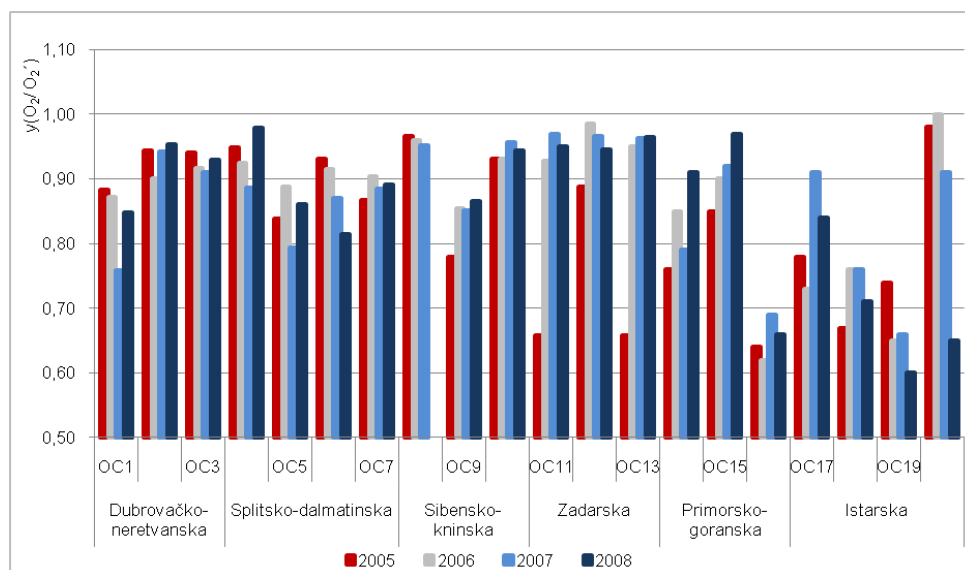
Slika 4.4. Udjeli zasićenja kisikom u pridnom sloju
