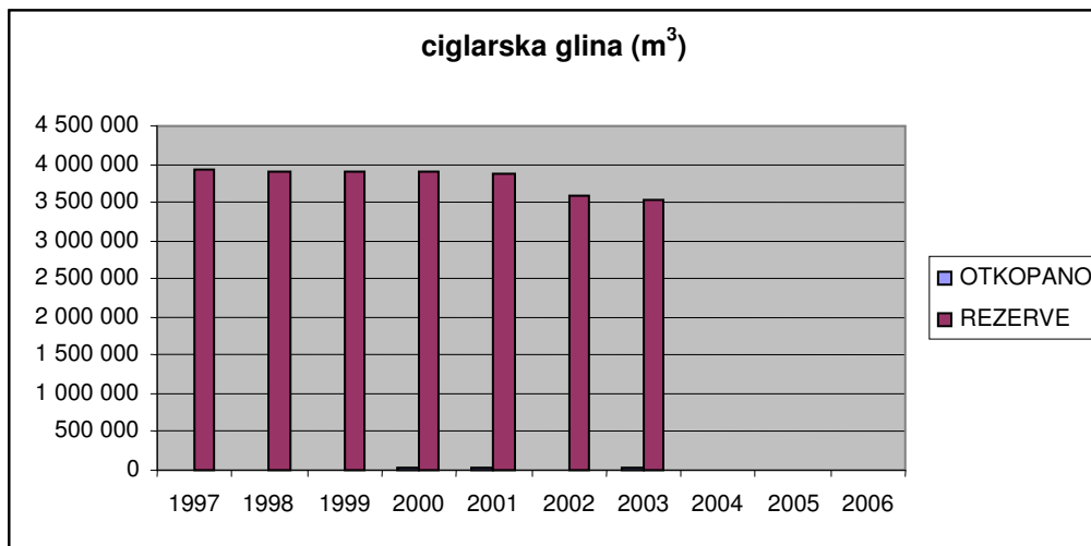
Prilog 5.12-2 Dijagramski prikaz rezervi i eksploatacije ciglarske gline, karbonatne sirovine za industrijsku preradu i tehničko-građevnog kamena u Brodsko-posavskoj županiji
