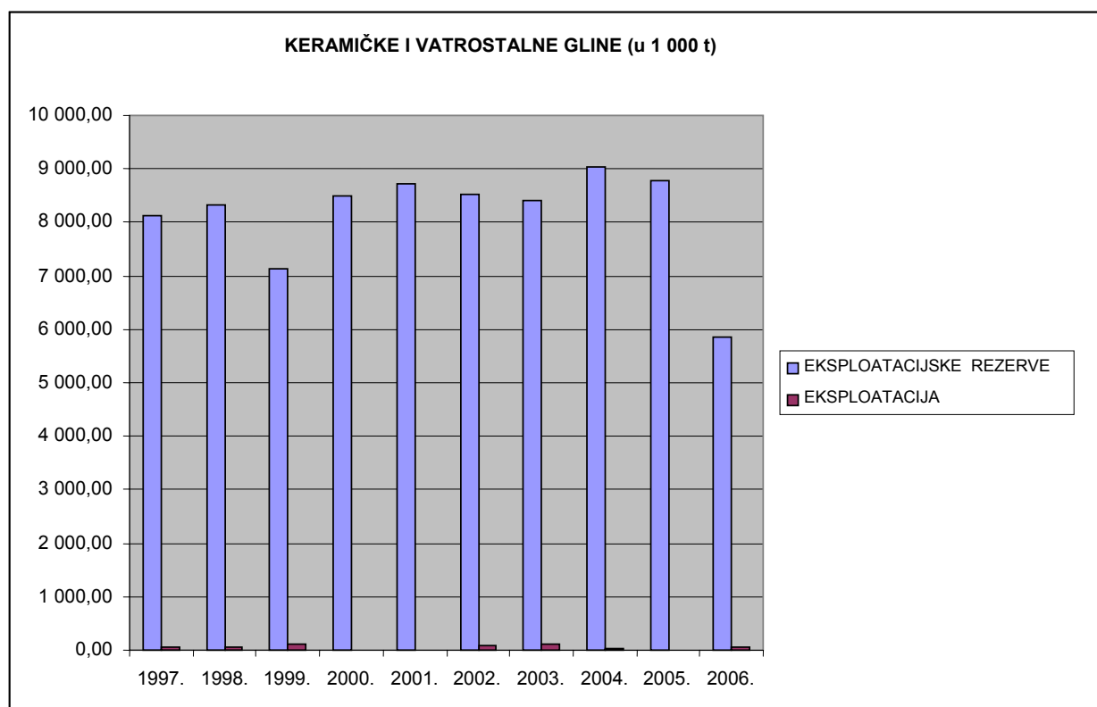
Slika 2.1-9 Eksploatacijske rezerve i eksploatacija keramičke i vatrostralne gline, za razdoblje 1997. – 2006. godina
