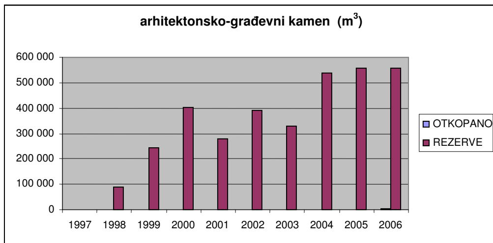
Prilog 5.19-2 Dijagramski prikaz rezervi i eksploatacije arhitektonsko-građevnog kamena i tehničko-građevnog kamena u Dubrovačko-neretvanskoj županiji
