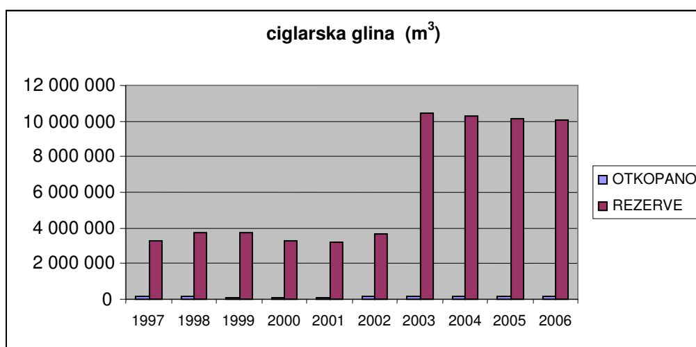
Prilog 5.5-2 Dijagramski prikaz rezervi i eksploatacije ciglarske gline, građevnog pijeska i šljunka i karbonatne sirovine za industrijsku preradu u Varaždinskoj županiji
