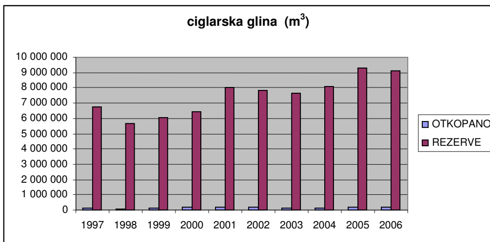
Prilog 5.16-2 Dijagramski prikaz rezervi i eksploatacije ciglarske gline u Vukovarsko-srijemskoj županiji
