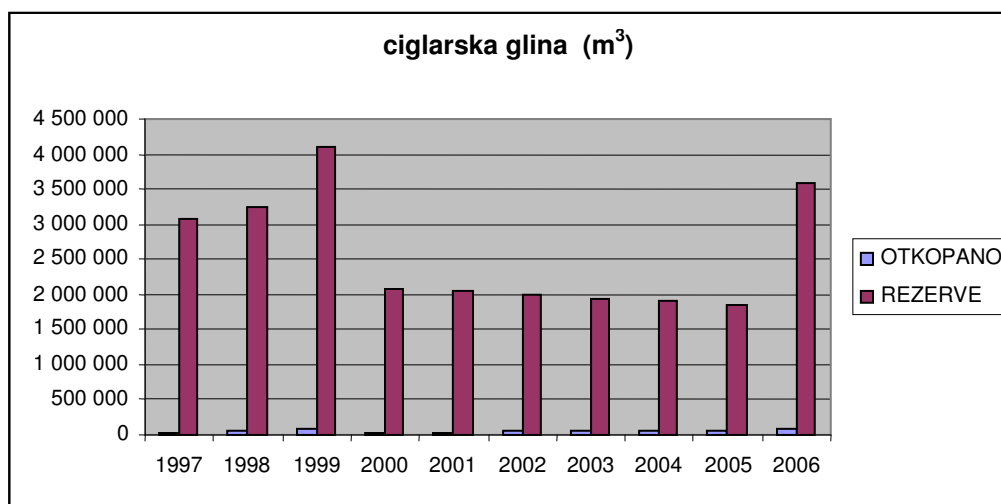
Prilog 5.7-2 Dijagramski prikaz rezervi i eksploatacije ciglarske gline, građevnog pijeska i šljunka i karbonatne sirovine za industrijsku preradu u Bjelovarsko-bilogorskoj županiji
