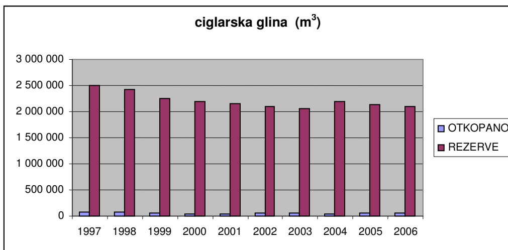
Prilog 5.20-2 Dijagramski prikaz rezervi i eksploatacije ciglarske gline i građevnog pijeska i šljunka u Međimurskoj županiji
