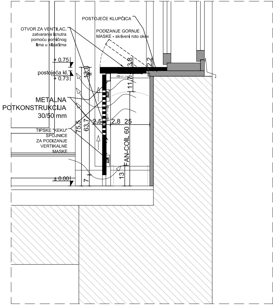
PRESJEK B-B
