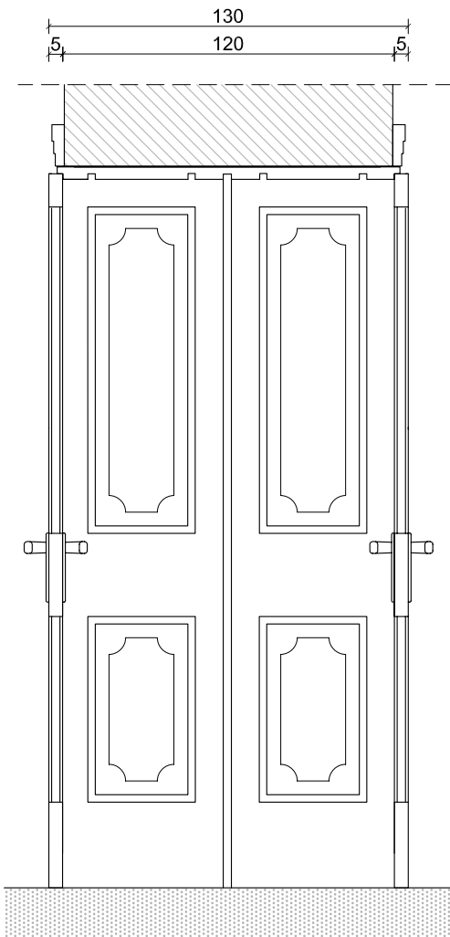
PRESJEK 1-1
