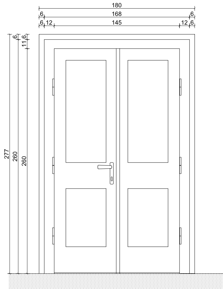
POGLED A-A ST-S18
