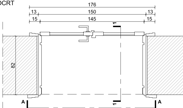
TLOCRT
