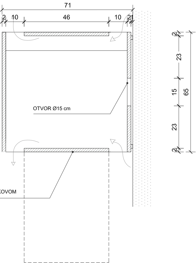
PRESJEK 1-1
