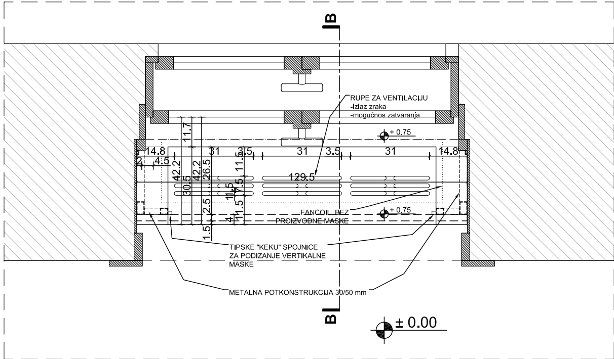
TLOCRT
