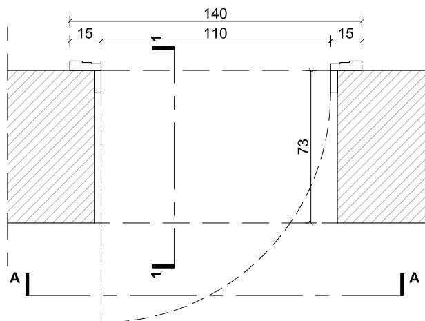
TLOCRT
